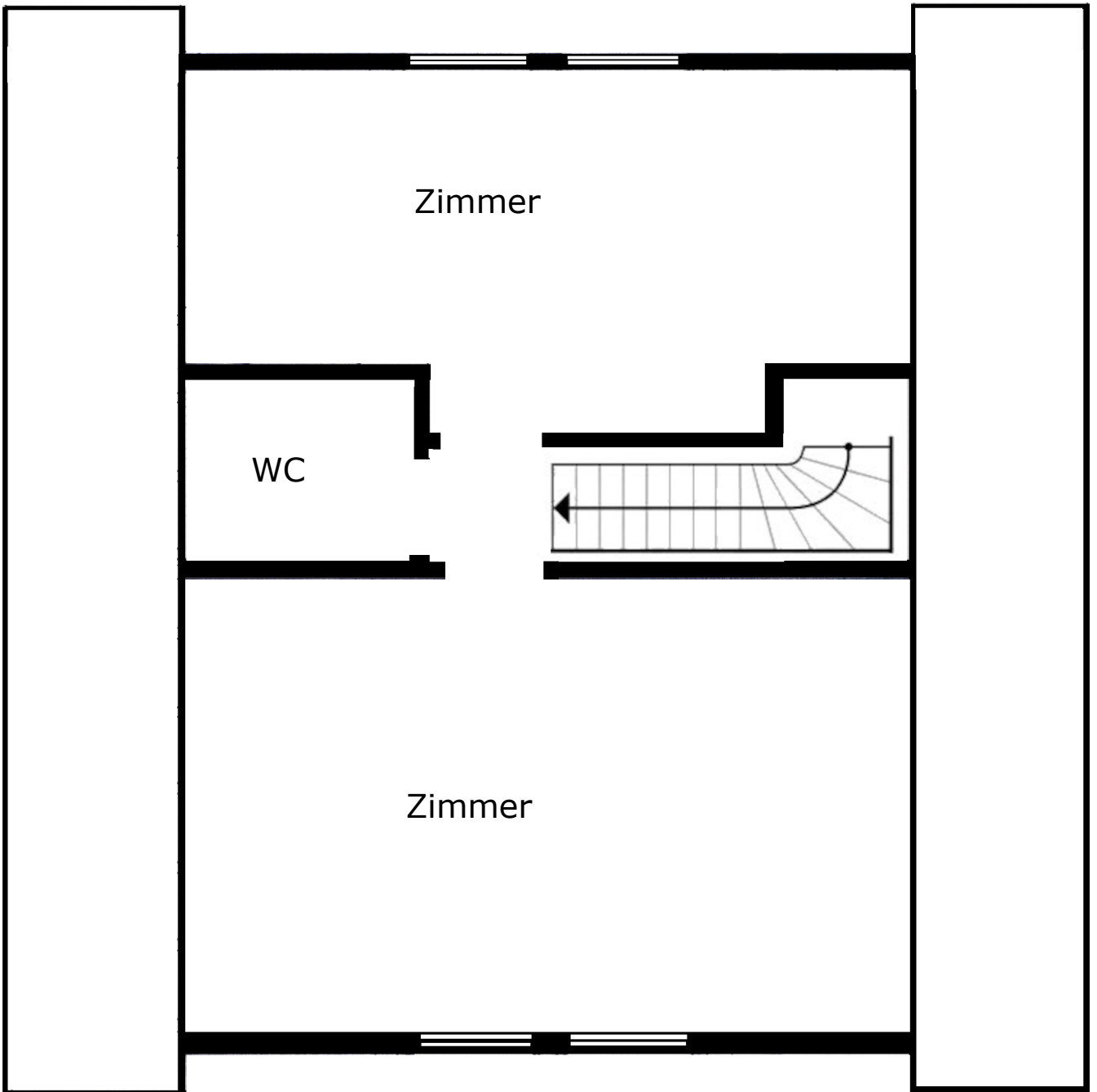
Grundriss Dachgeschoss
